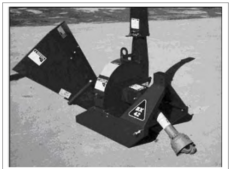
Fig. 9 DISCHARGE CHUTE
