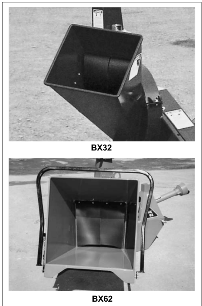
Fig. 31 CURTAIN
